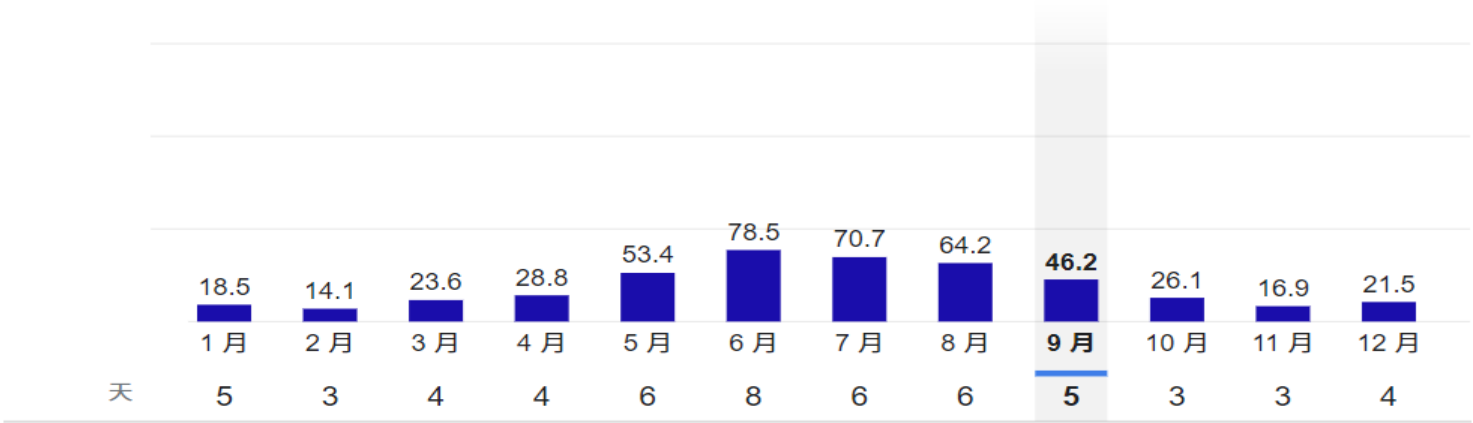
降雪量 (毫米)
