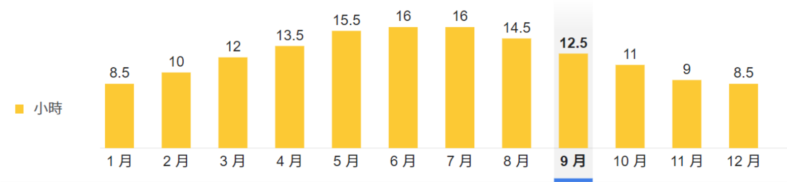
日照時數
